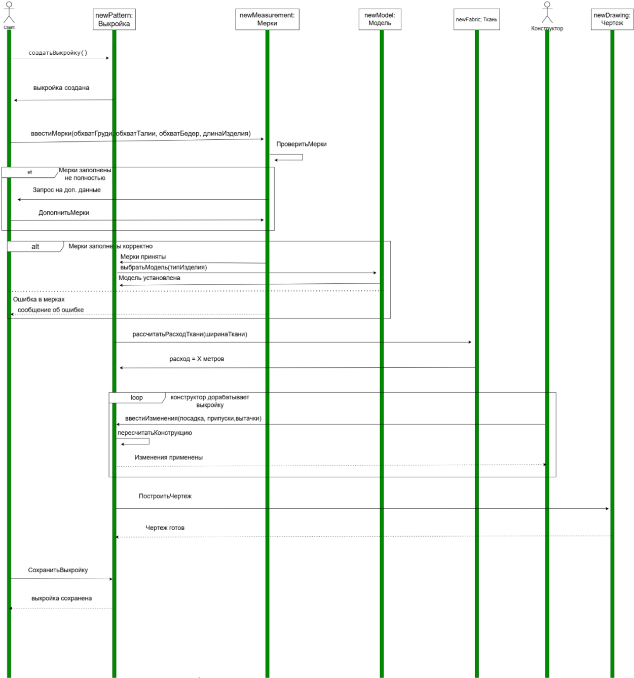
Диаграмма последовательности
